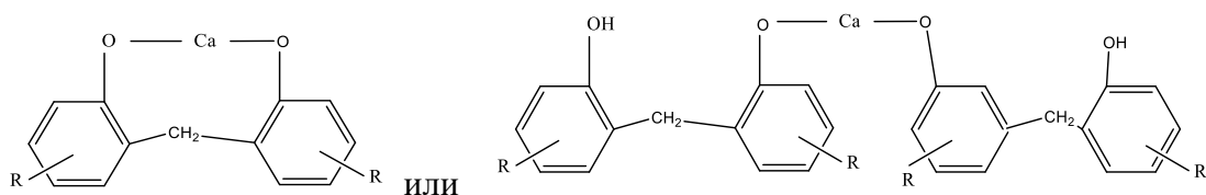
Рис. 1. Конденсированные формальдегидом алкилфеноляты кальция
