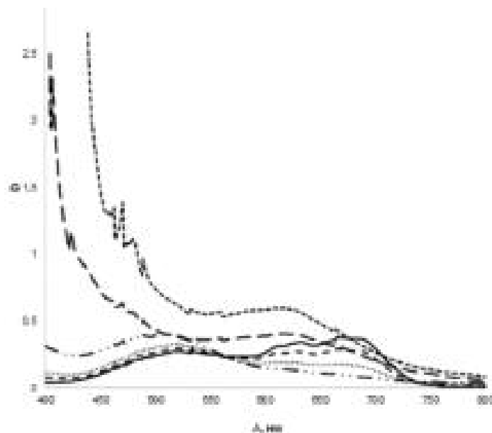
Рис. 2. Зависимость оптической плотности D от длины волны \lambda
