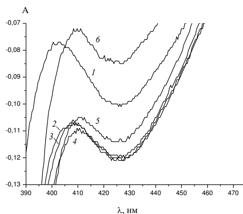
Рис. 4. Спектры поглощения карбонилксиды ФМ. CH_3CN , 343 К. [ЭС]_0 = 1.04 , [ТСК] = 0.093 , [Py] = 0.4 моль/л. Время: 1200, 1800, 2400, 3000, 3600, 4200 с.
