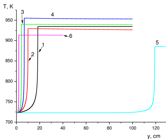
Рис. 1. Расчет распределения температуры по длине реактора при использовании кинетических моделей Веденеева (1), Ranzi (2), NUI Galway (3), Battin-Leclerc (4), Rasmussen (5) и Lodeng (6). Метано-воздушная смесь с начальным отношением [O_2]_0/[CH_4]_0=0.05 , p=80 атм и начальной температурой 723 К.
