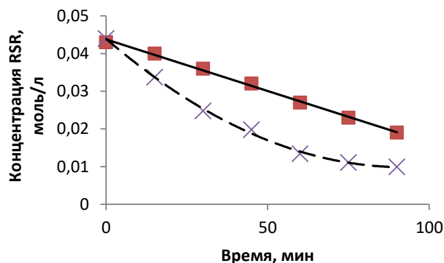
Рис. 3. Зависимость концентраций RSR от времени в экспериментах, проводимых в различное время.
