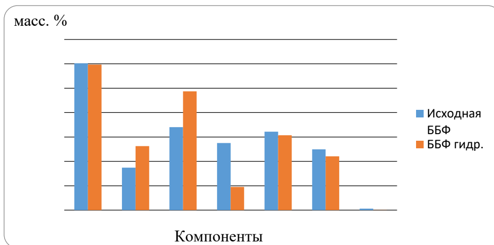
Рис. 1. Компонентный состав фракции С4-С5 в составе ББФ до и после гидрирования (1- изобутан; 2 - н-бутан; 3 - транс-бутен-2; 4 - бутен-1; 5 - изобутен; 6 - цис-бутен-2; 7 – 3метилбутен-1)
